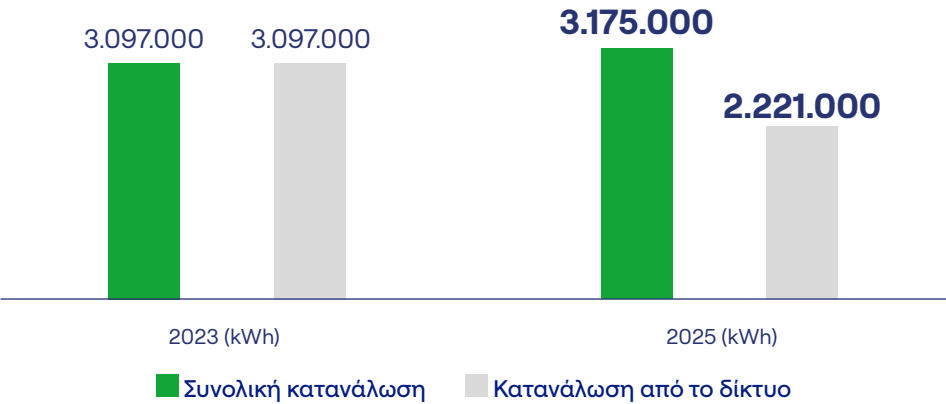
Σχήμα 1: Σύγκριση της συνολικής κατανάλωσης ηλεκτρικής ενέργειας και της κατανάλωσης από το δίκτυο πριν και μετά την εγκατάσταση του φωτοβολταϊκού συστήματος (2023–2025)
